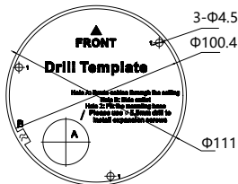
Рисунок 2-3 Шаблон крепления
