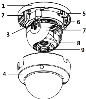
Рисунок 1-1 Купольная камера (1)
